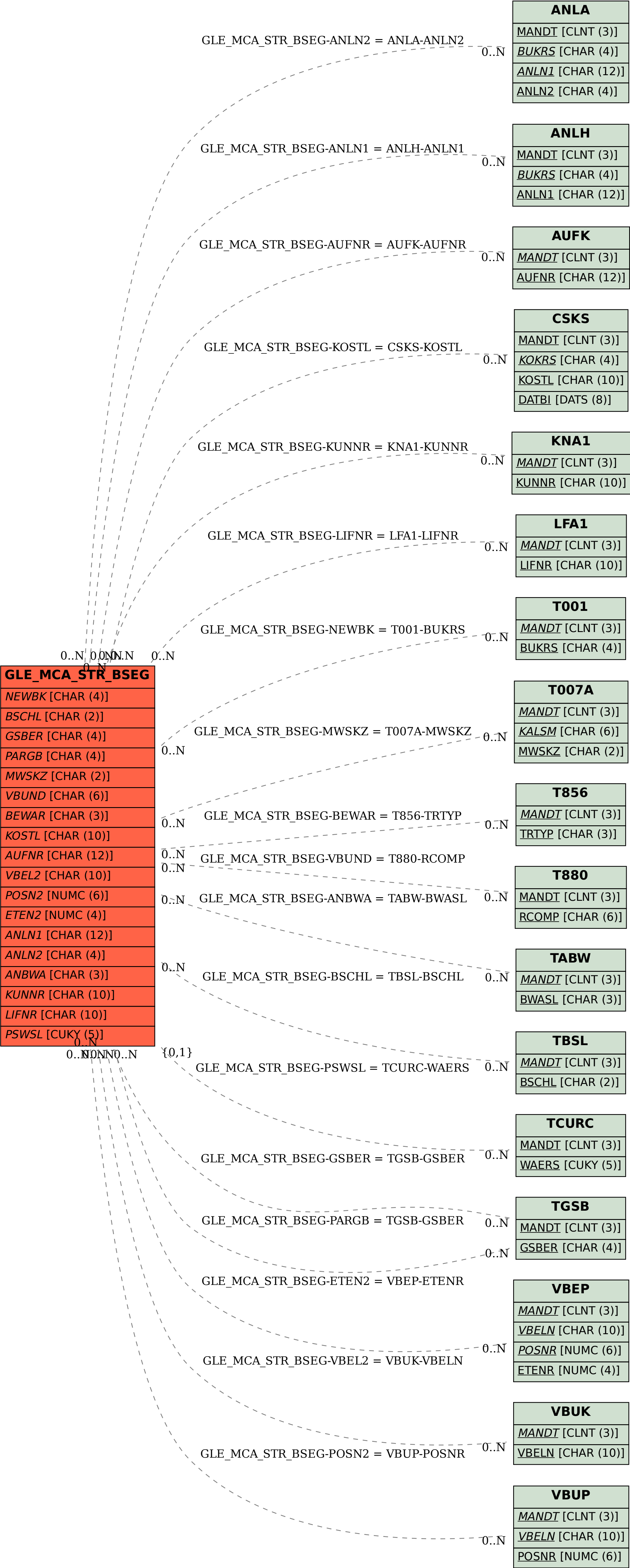
SAP ABAP table GLE_MCA_STR_BSEG {MCA STR BSEG}
