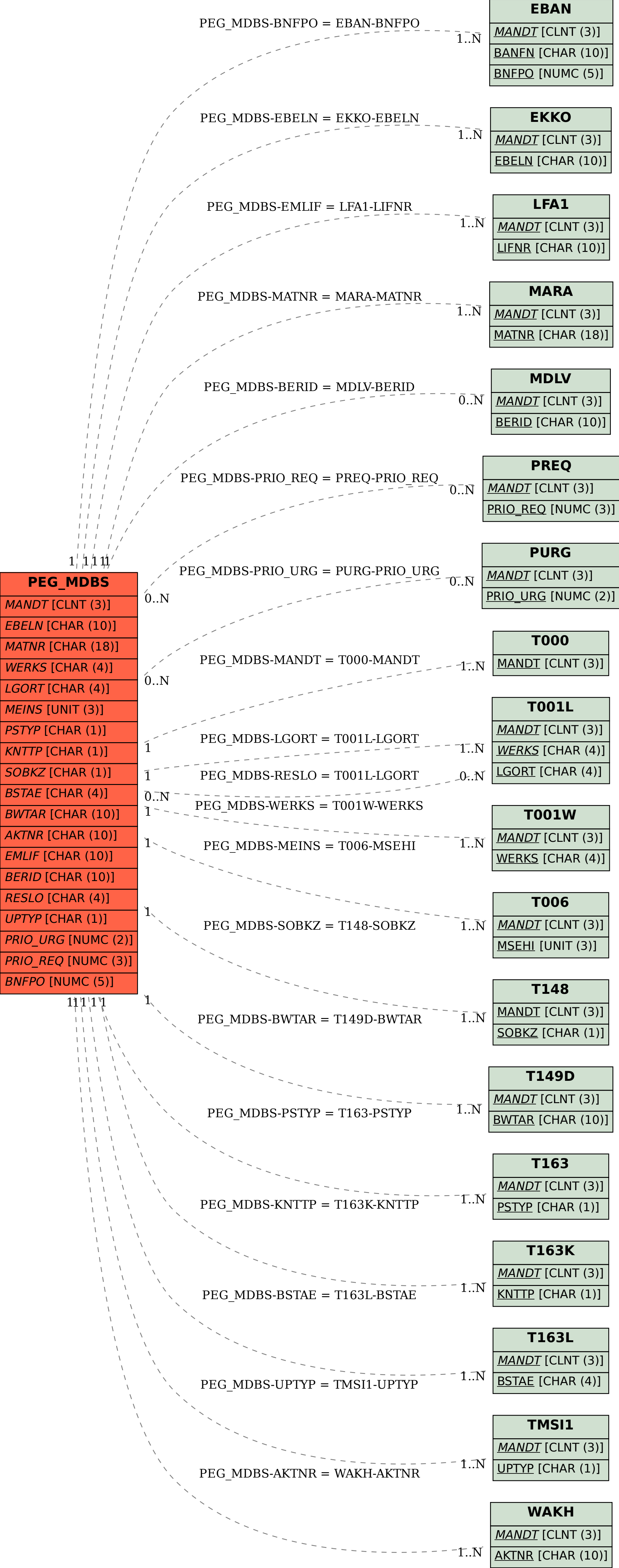
SAP ABAP table PEG_MDBS {PEG_MDBS}
