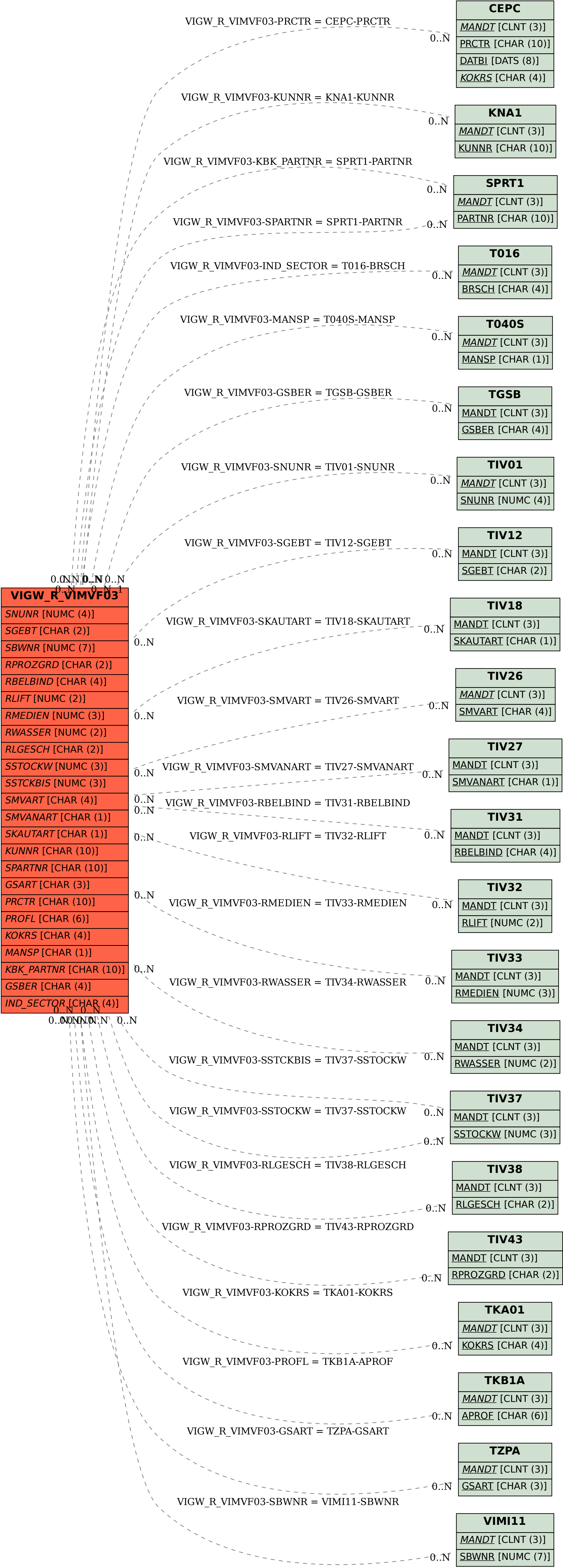
SAP ABAP table VIGW_R_VIMVF03 {Immobilien gew.: Mieteinheiten / Mietvertrag}
